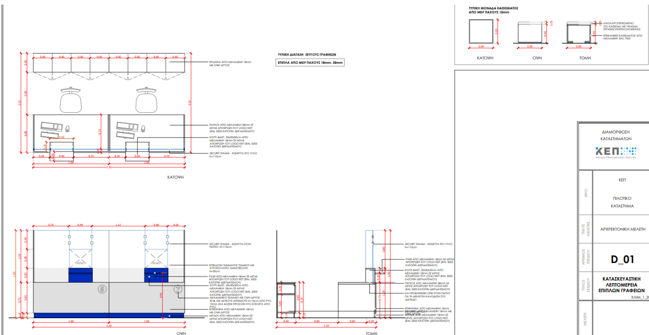
Σχέδιο D_01
